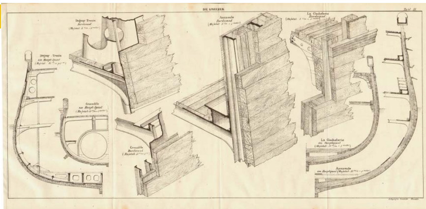
Presjek broda i dijelovi krstarice, Pola, 1876.
